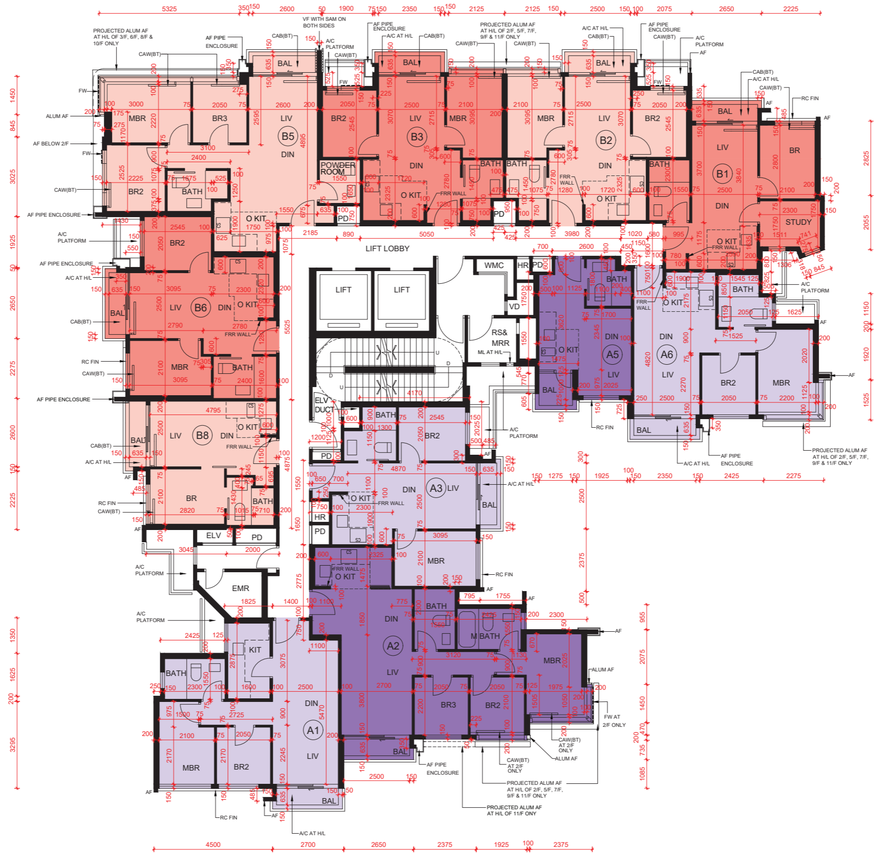
GREENWOOD TOWER 2 2/F-3/F AND 5/F-11/F FLOOR PLAN 翠景閣第2座 2樓至3樓 及 5樓至11樓平面圖
